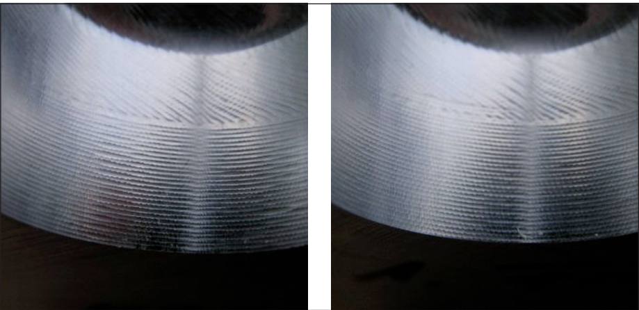
图8：机床振动对工件表面的影响： 8a：无加加速平滑处理，Z轴振动导致表面划伤 8b：iTNC 530系统的运动控制功能有效避免了振动导致的表面质量问题
