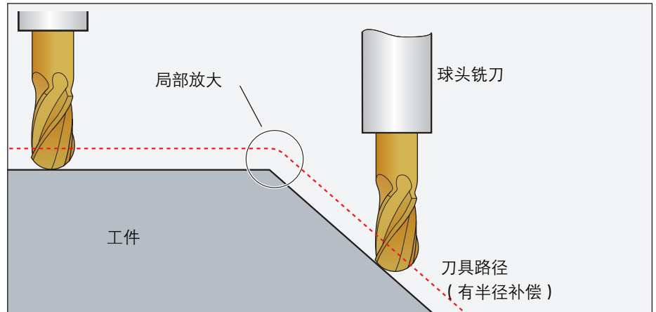
图2：球头铣刀TCP刀具路径
