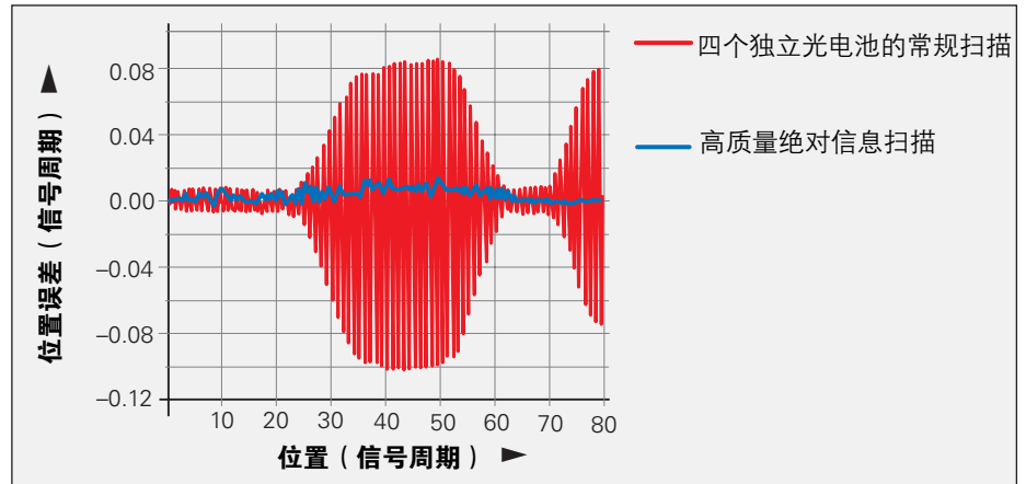
污染对位置精度影响（典型测量值）
