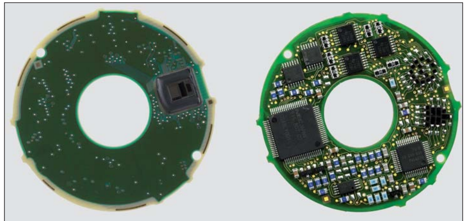
高质量扫描型绝对式旋转编码器的PCB板（opto-ASIC）和四个光电池扫描的PCB板
